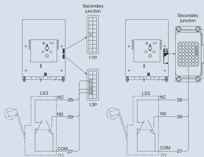
Fig. 71 Wiring diagram
